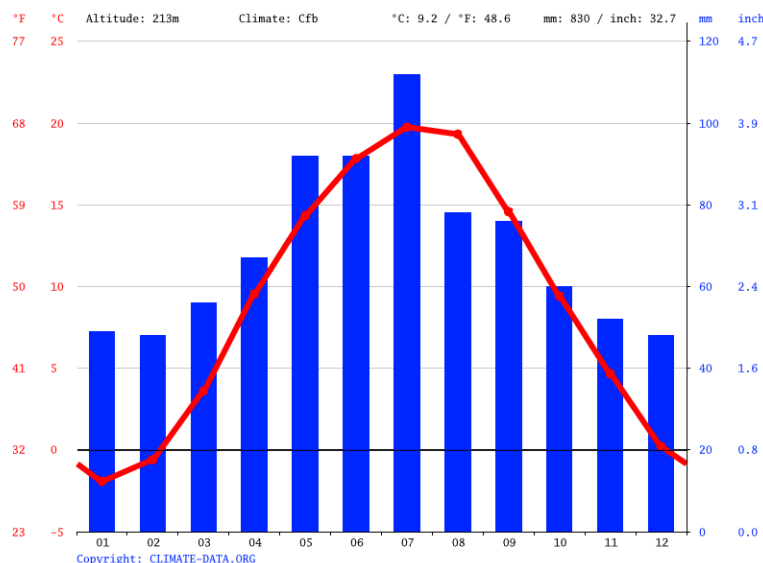
Ryc. Wykres klimatyczny miasta Czechowice-Dziedzice
